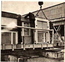
Fot. 5. Ładowanie gotowych elementów do pojemnika
